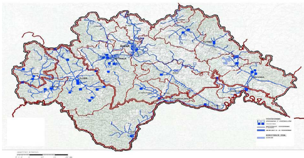
Slika 4. Vodoopskrbna mreža na području SMŽ iz koje je vidljiva vodoopskrbna mreža LAG-a 2
